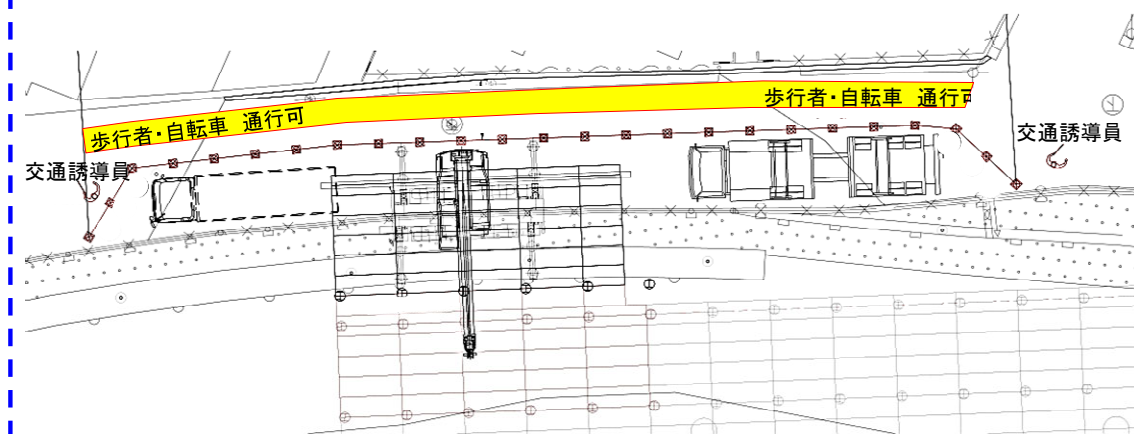
交通規制工程表
